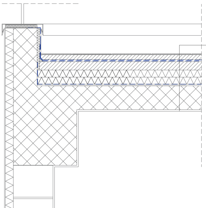
ДЕТАЛ НА ПАРАПЕТ
