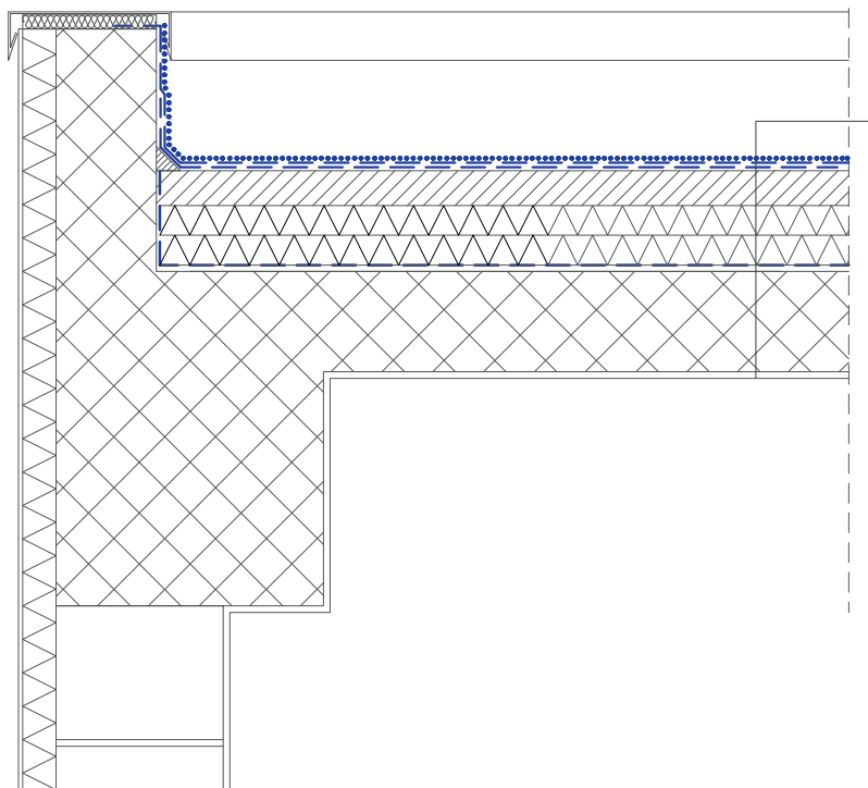
ДЕТАЛ НА ПАРАПЕТ
