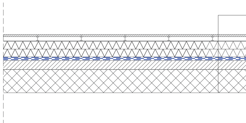
РАМЕН ИНВЕРЗЕН ПРООДЕН КРОВ - систем на хидроизолација со завршен слој од плочки поставени на носачи
