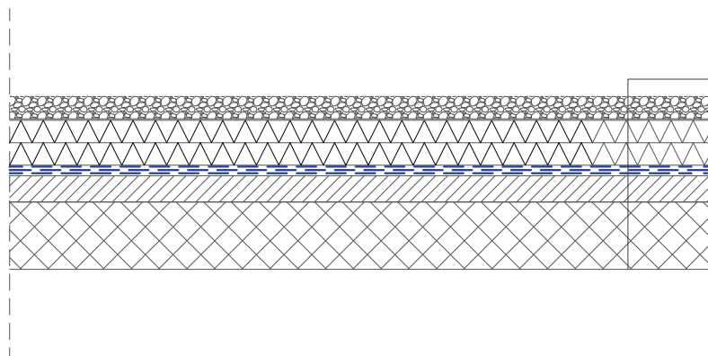
РАМЕН ИНВЕРЗЕН НЕПРООДЕН КРОВ - систем на хидроизолација со завршен слој од шљунак
